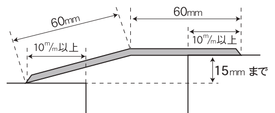
への字タイプ120巾の施工断面図
