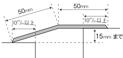
への字タイプ100巾の施工断面図
